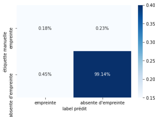
Figure 4. Matrice de confusion après redressement statistique de l'échantillon annoté
