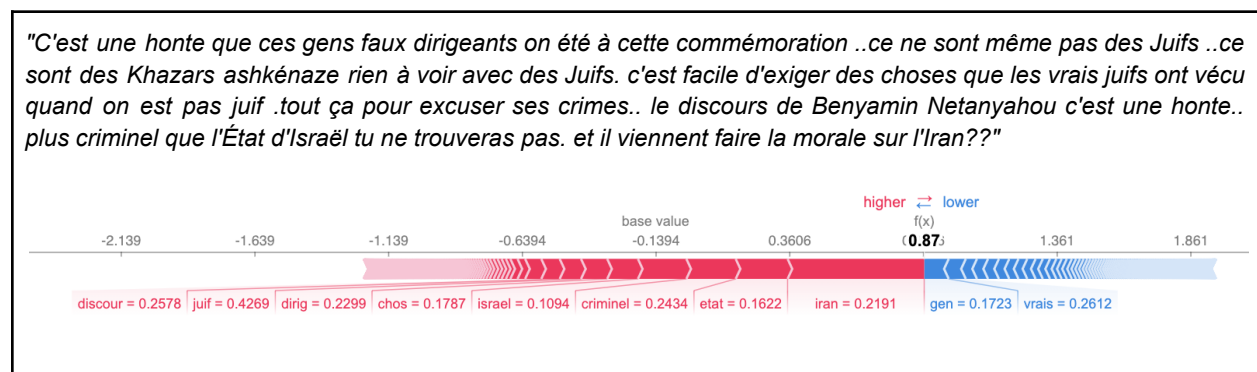
Fig 7 - « Diagramme de force » montrant le fonctionnement de l'algorithme tf-idf appliqué sur un commentaire. En rouge, les mots qui contribuent à l'empreinte antisémite du commentaire et en bleu ceux qui n'y contribuent pas.
